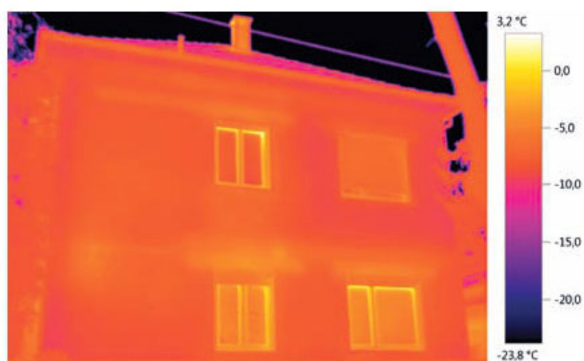
Термограмма без функции testo ScaleAssist
